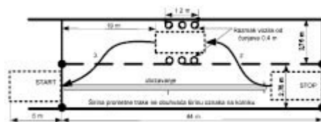
Slika 5. Prometno-tehnički element za vožnju unaprijed-unatrag s promjenom smjera za vozila B kategorije
