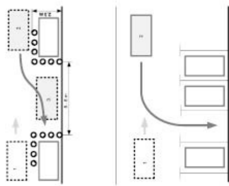
Slika 7. Prometno-tehnički element za parkiranje vozila B kategorije
